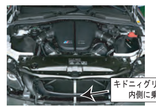
19: エアフロセンサーのカバーを取り付けます。バンパーを元の通り取り付けます。*導入ダクト先端部はキドニイグリル内側に乗るような配置になります。
