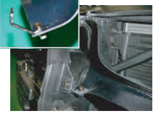
14: 導入ダクトにステア(T-0311A)を左右同様に取り付けます。両サイドをビスA、ナットを使用して固定します。
