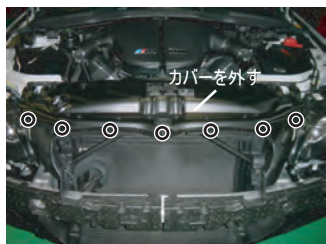
4: バンパーを取り外します。ラジエーター上部のカバーを外し、○印のボルトを外し、バンパーを取り外します。(トルクスボルト7ヶ所)
