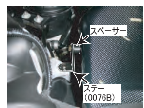
17: 右側のダクトを固定します。ステアとダクトの間にスペーサーを挟みビスCで固定。ボディ側はビスBで固定。
