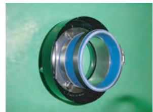
10: エアフロアダプター、整流ハニカムとラバーホースの間にフィルターケースを挟み組み付けます。ハニカムは金属メッシュがエンジン側です。
