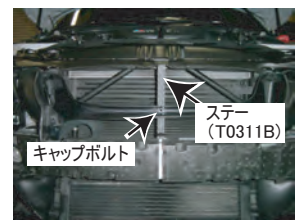
13: 導入ダクトのセンター部固定用のステア(T0311B)を取り付けます。ステア上側はバンパーと共締めします。下側はバンパーフレームと発泡スチロールの間に挟みます。
