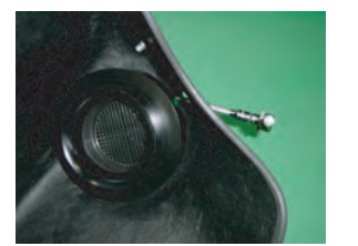
11: グロメットを外し、サービスホールからドライバーを入れてホースバンドを締め付け、固定します。ラバーホースとエアフロは互いに押し付け、フィルターケースと密着させた状態でバンドで締めます。固定後は元の通り、グロメットで塞いでください。
