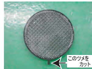
8: 取り出した整流ハニカムのツメをカットします。
